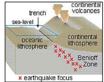
Wadati-Benioff zone
